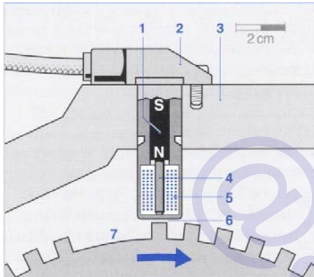
شکل ۵-۱: حسگر سرعت موتور
