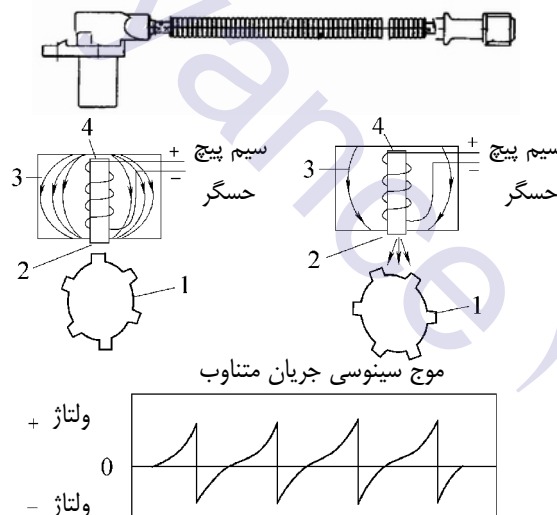
شکل ۵-۲: اصول عملکرد حسگر سرعت موتور
