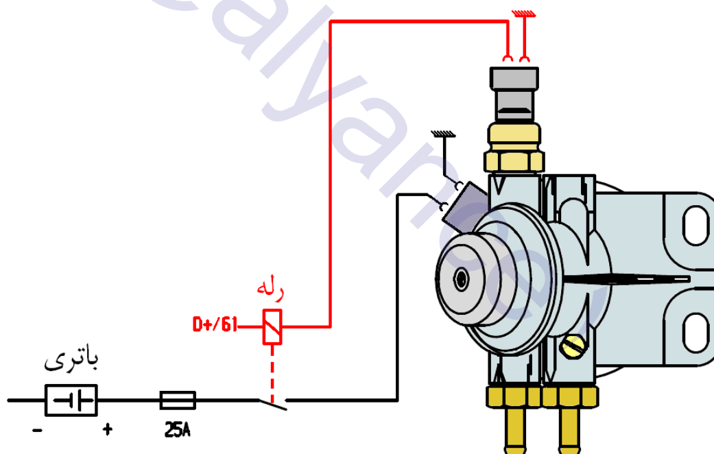
شکل ۵-۱۳ مدار فرمان (تحریک) رله گرمکن سوخت
